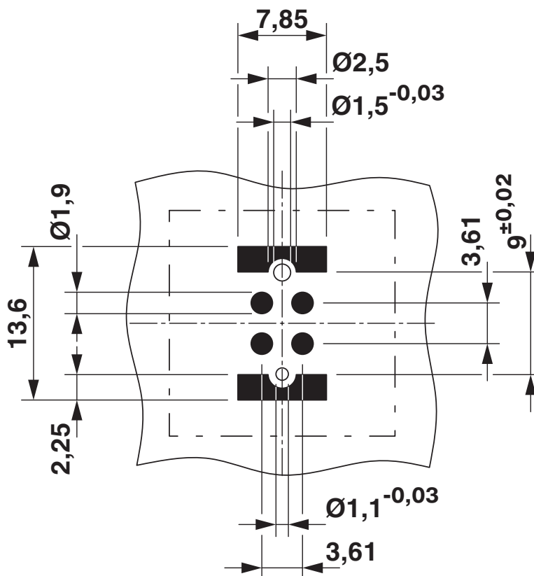
Otworowanie/geometria płytek lutowniczych
