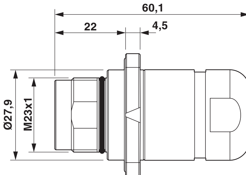
Rysunek wymiarowy
