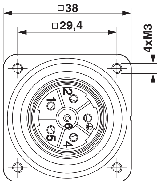
Rysunek wymiarowy
