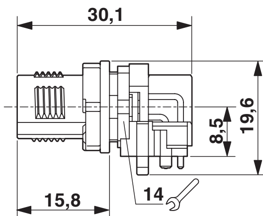
Rysunek wymiarowy
