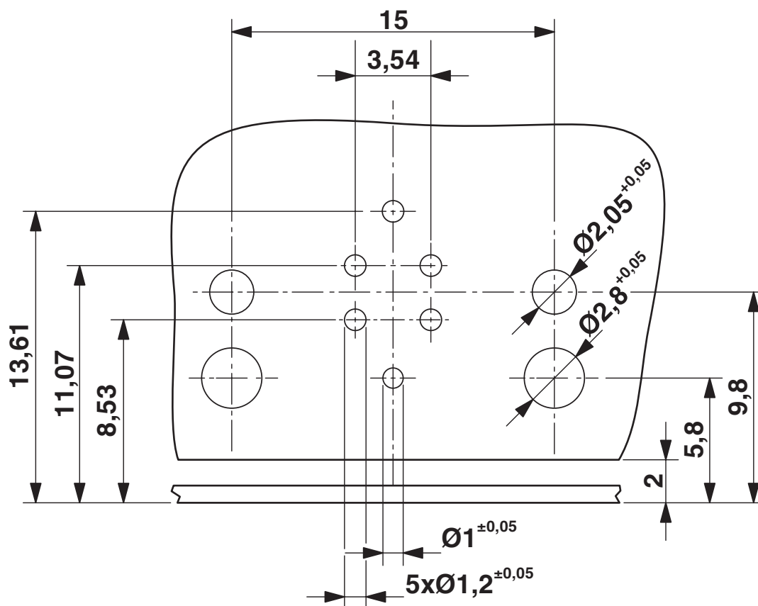
Otworowanie/geometria płytek lutowniczych
