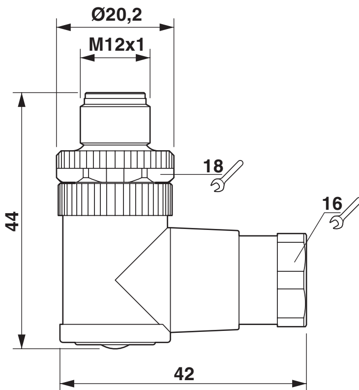
Rysunek wymiarowy
