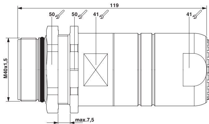
Rysunek wymiarowy
