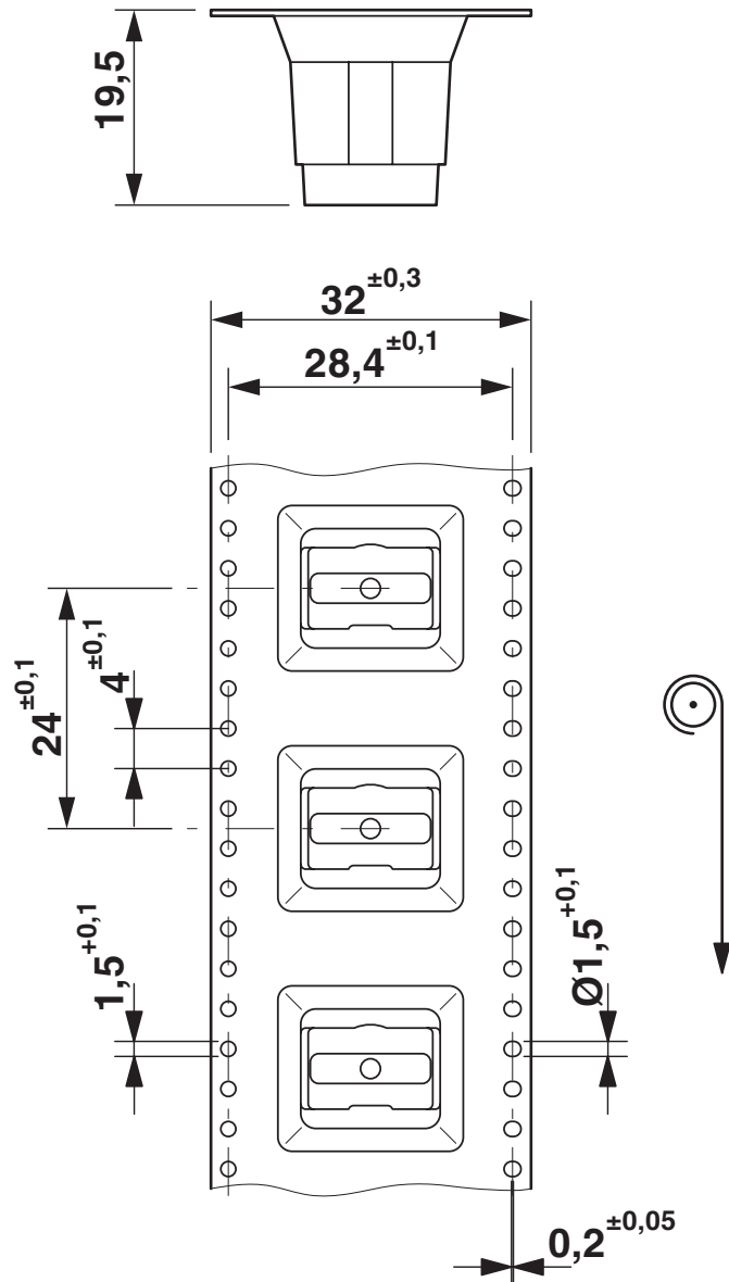
Rysunek wymiarowy
