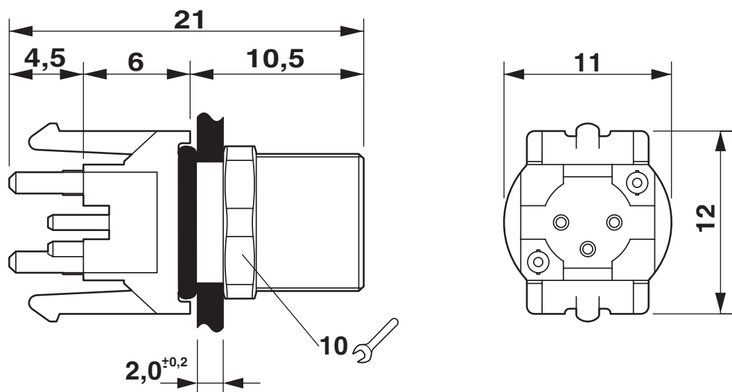
Rysunek wymiarowy
