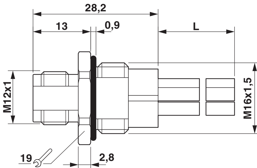
Rysunek wymiarowy
