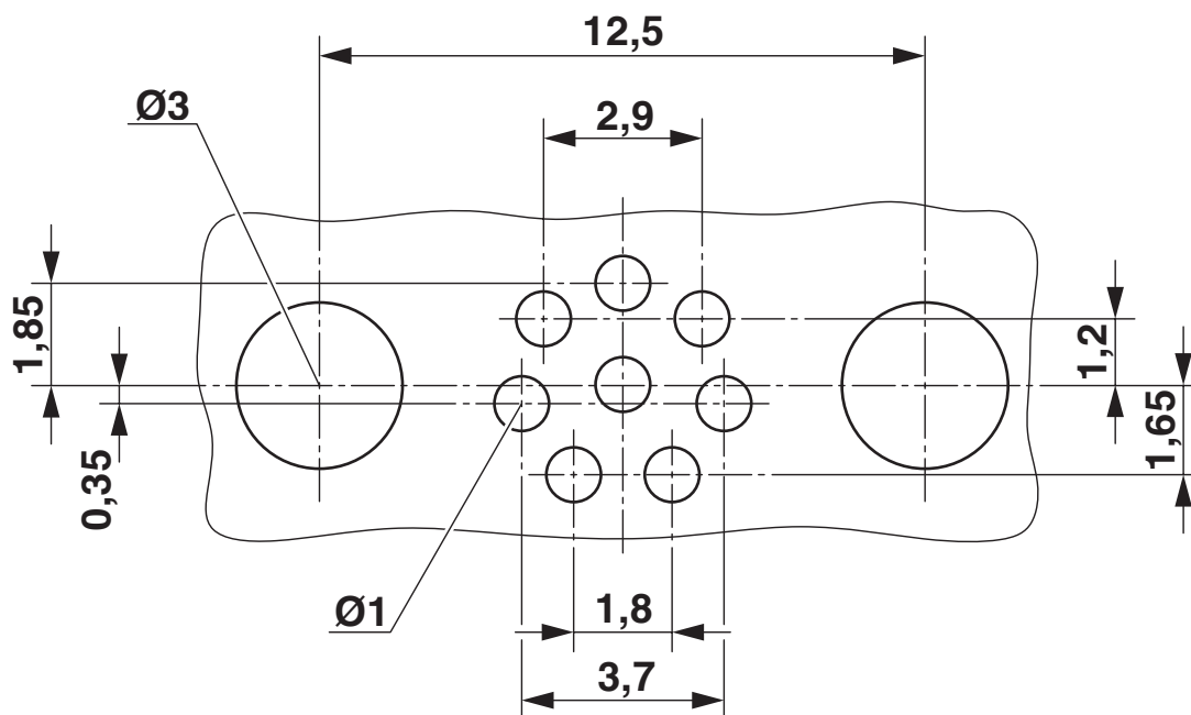
Schemat otworów we wtyku
