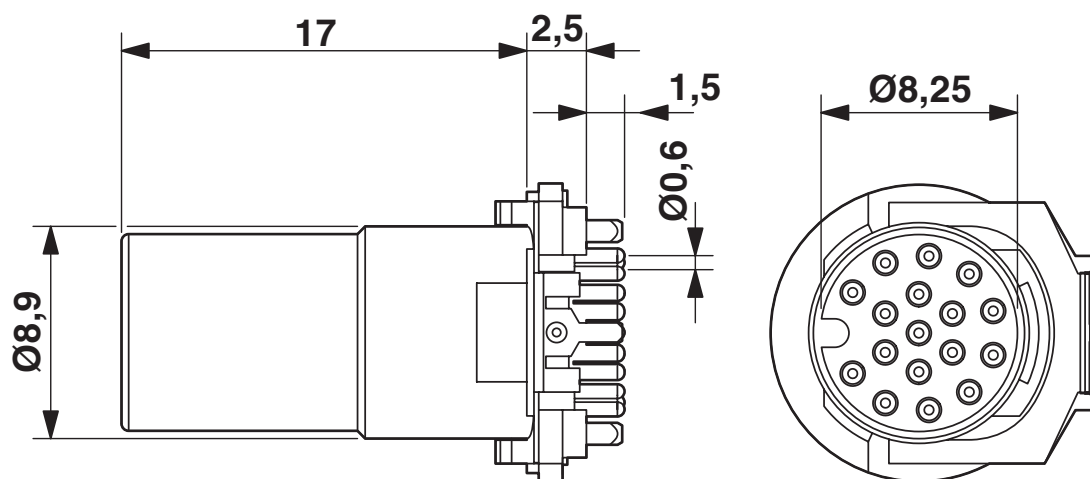
Rysunek wymiarowy
