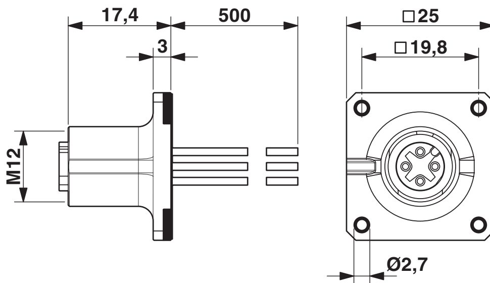
Rysunek wymiarowy
