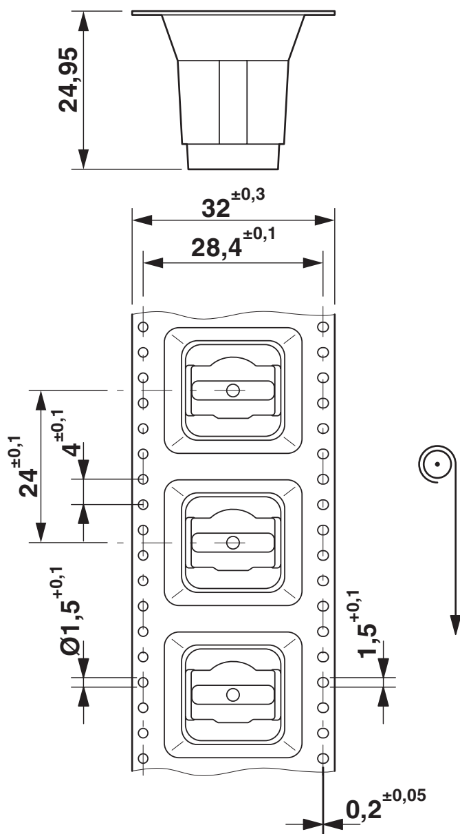
Rysunek wymiarowy
