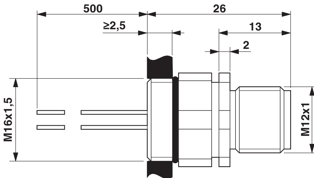
Rysunek wymiarowy
