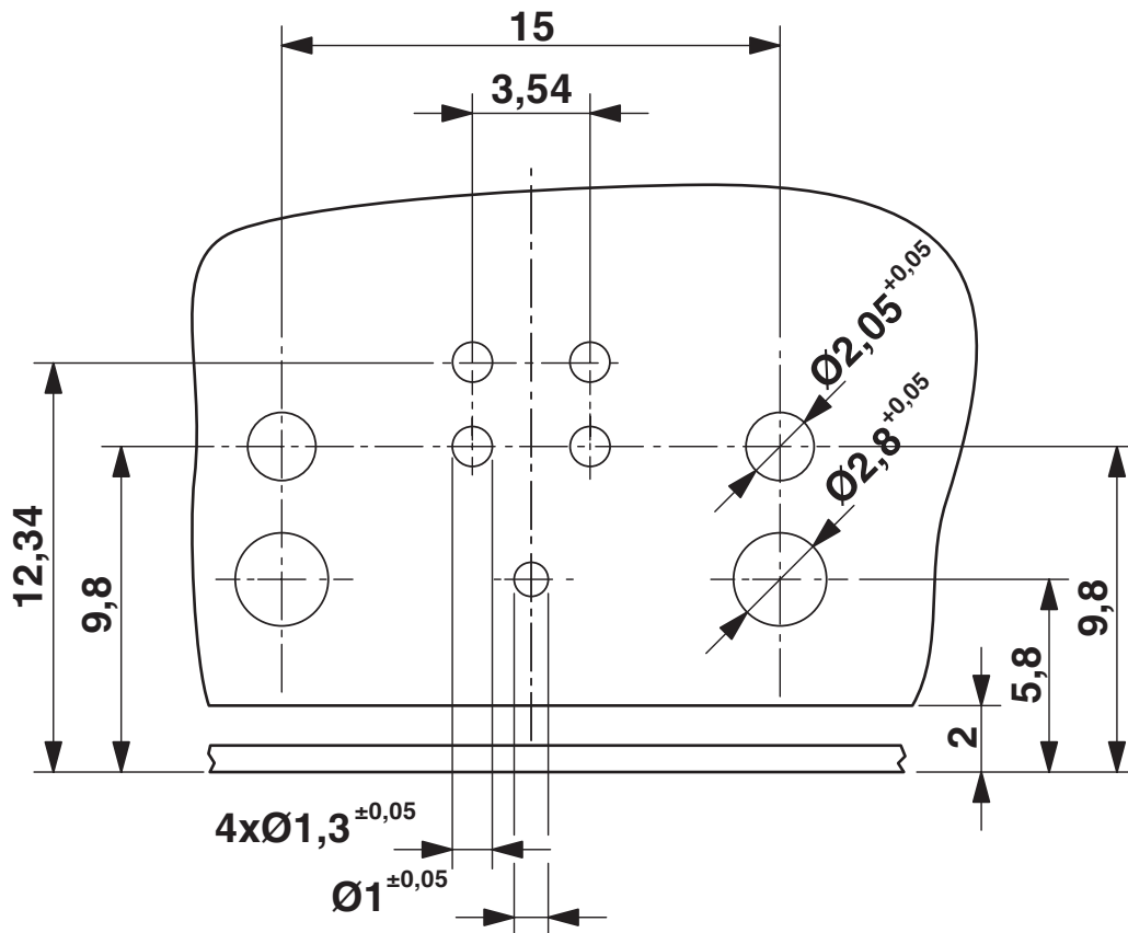
Rysunek wymiarowy
