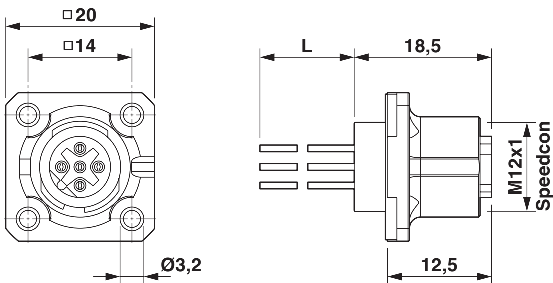
Rysunek wymiarowy
