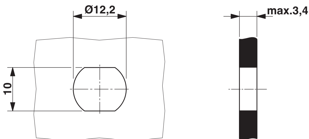
Rysunek wymiarowy
