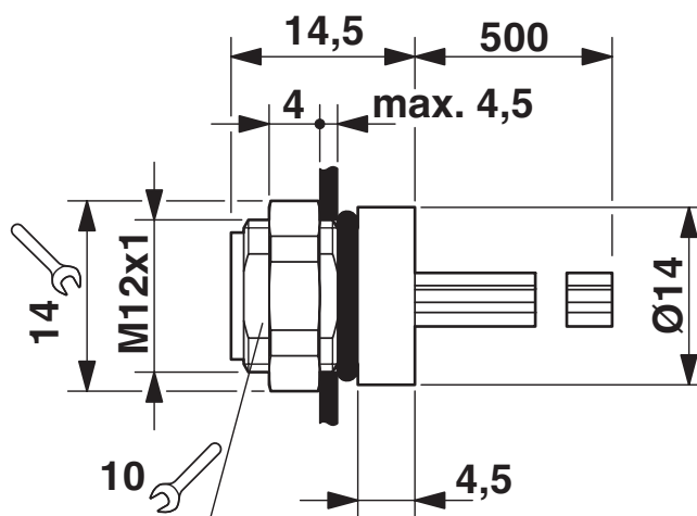
Rysunek wymiarowy
