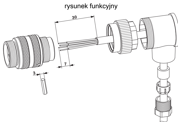
Rysunek schematyczny
