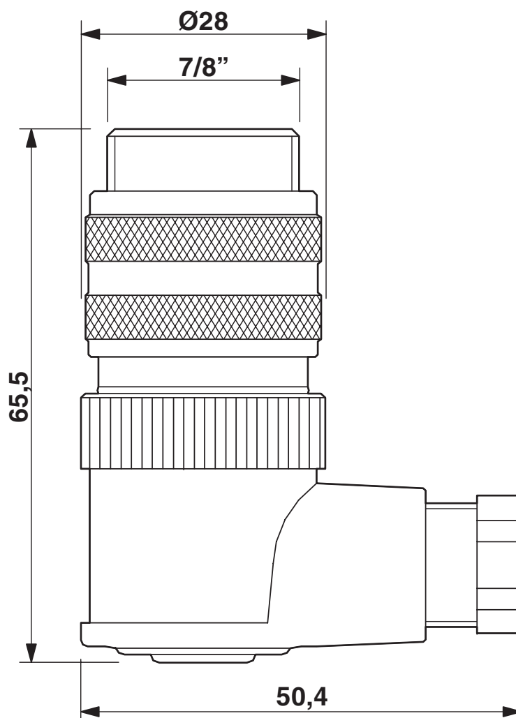
Rysunek wymiarowy
