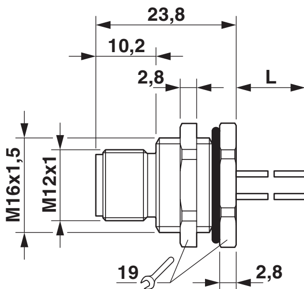
Rysunek wymiarowy
