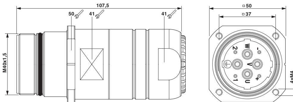
Rysunek wymiarowy
