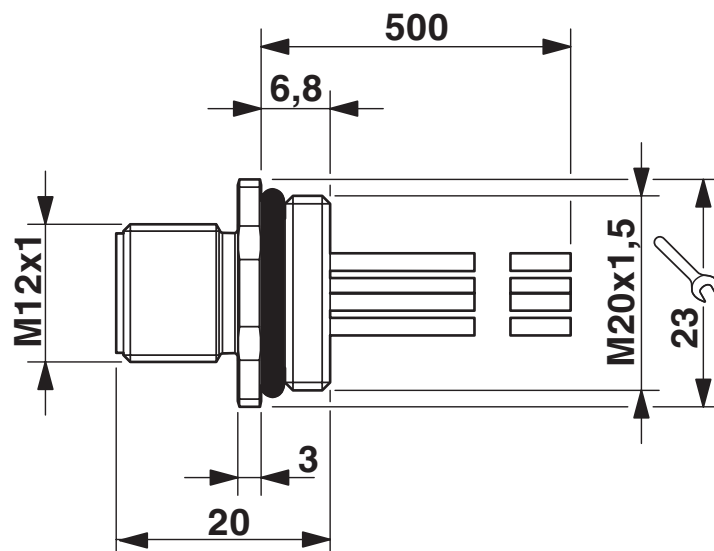
Rysunek wymiarowy
