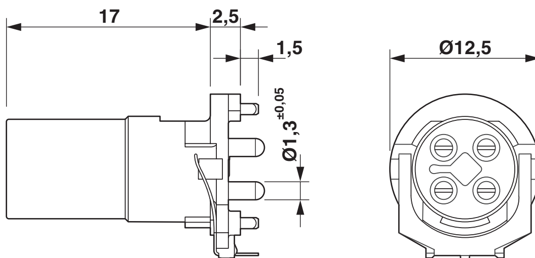
Rysunek wymiarowy
