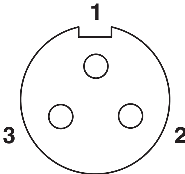
Układ styków, gniazdo 7/8" 16UNF, 3-biegunowe, widok od strony gniazda
