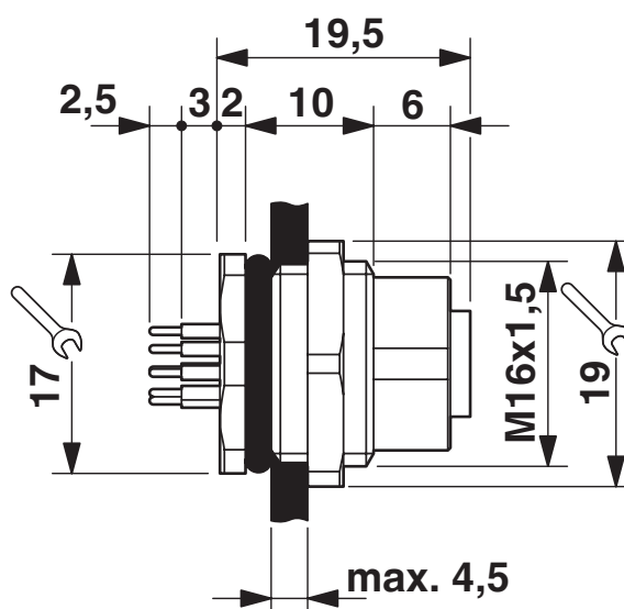
Rysunek wymiarowy
