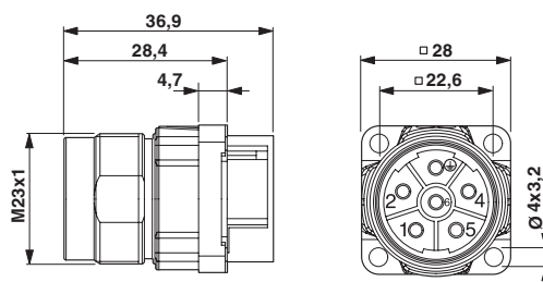
Rysunek wymiarowy
