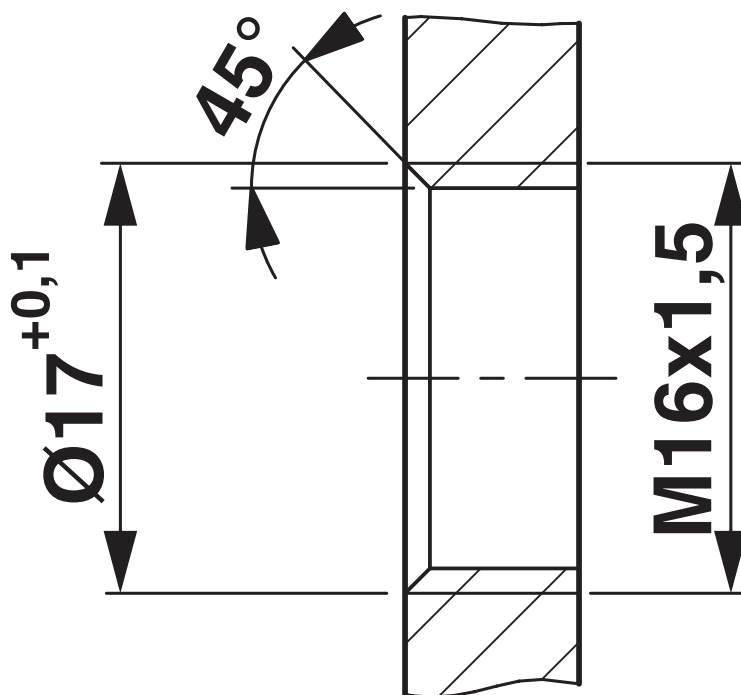
Fragment obudowy dla gwintu mocującego M16, ściana montażowa z gwintem
