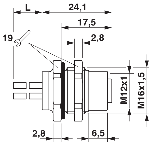
Rysunek wymiarowy
