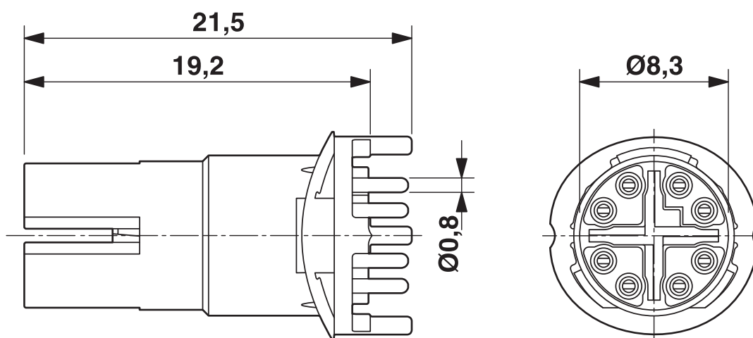
Rysunek wymiarowy
