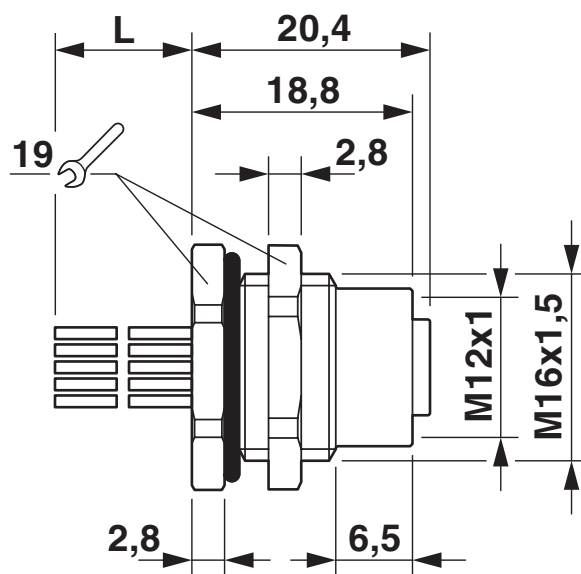
Rysunek wymiarowy
