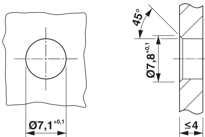
Rysunek wymiarowy
