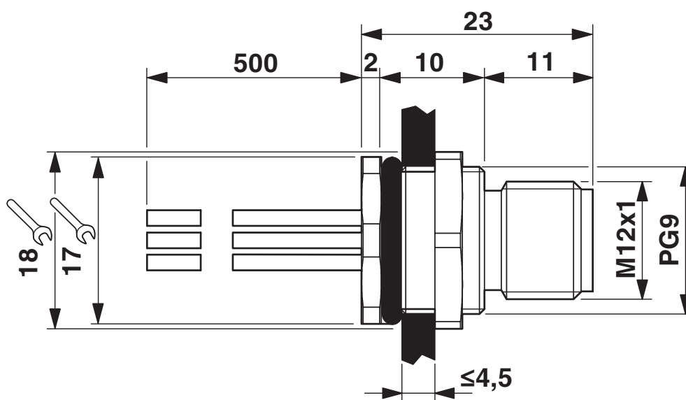
Rysunek wymiarowy
