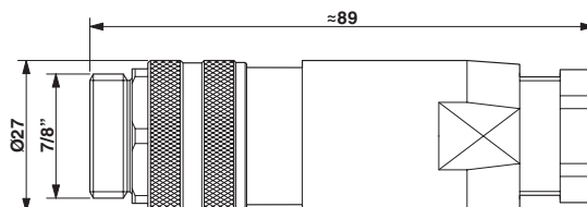
Rysunek wymiarowy
