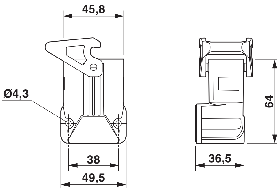
Rysunek wymiarowy
