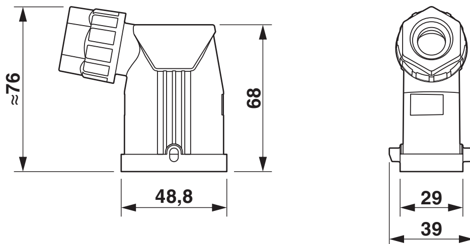
Rysunek wymiarowy
