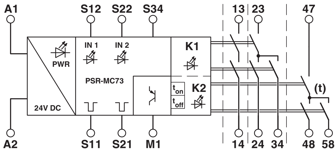
Schemat blokowy
