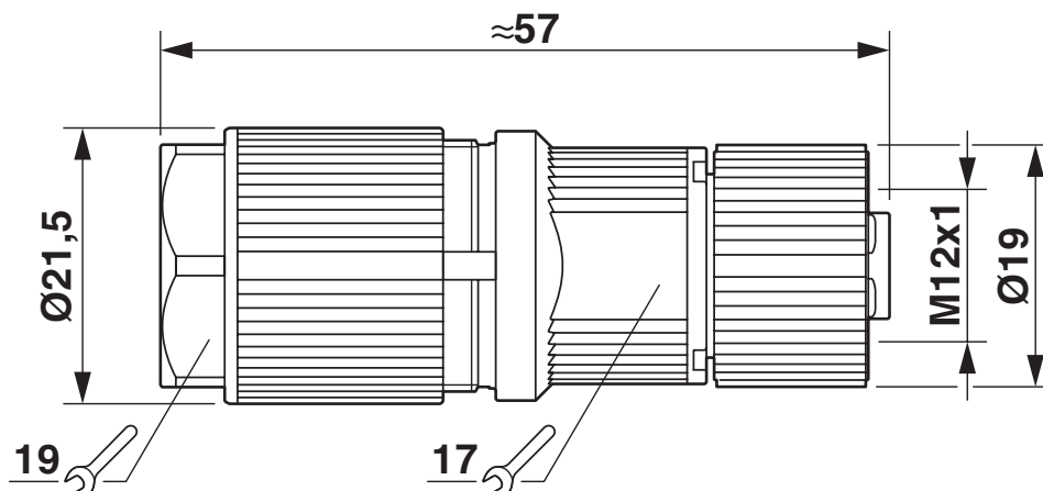
Rysunek wymiarowy
