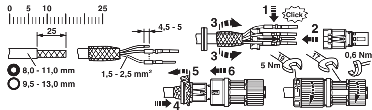
rysunek funkcyjny
