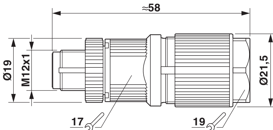
Rysunek wymiarowy
