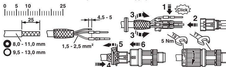
rysunek funkcyjny
