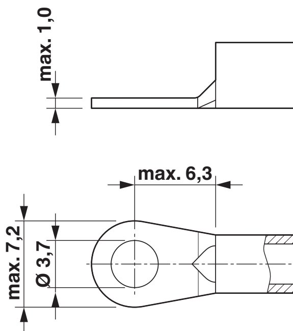
Rysunek wymiarowy
