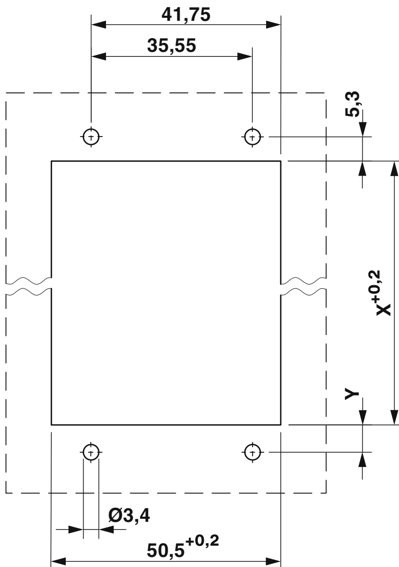
Rysunek wymiarowy
