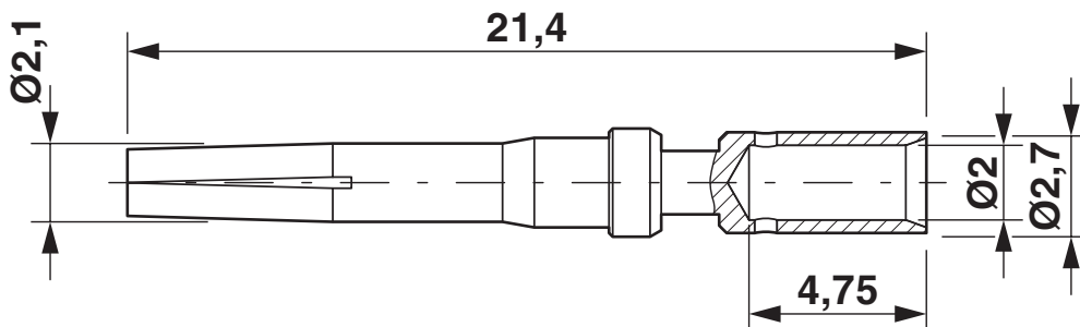
Rysunek wymiarowy
