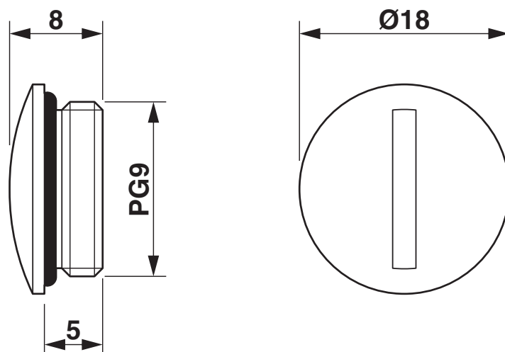
Rysunek wymiarowy
