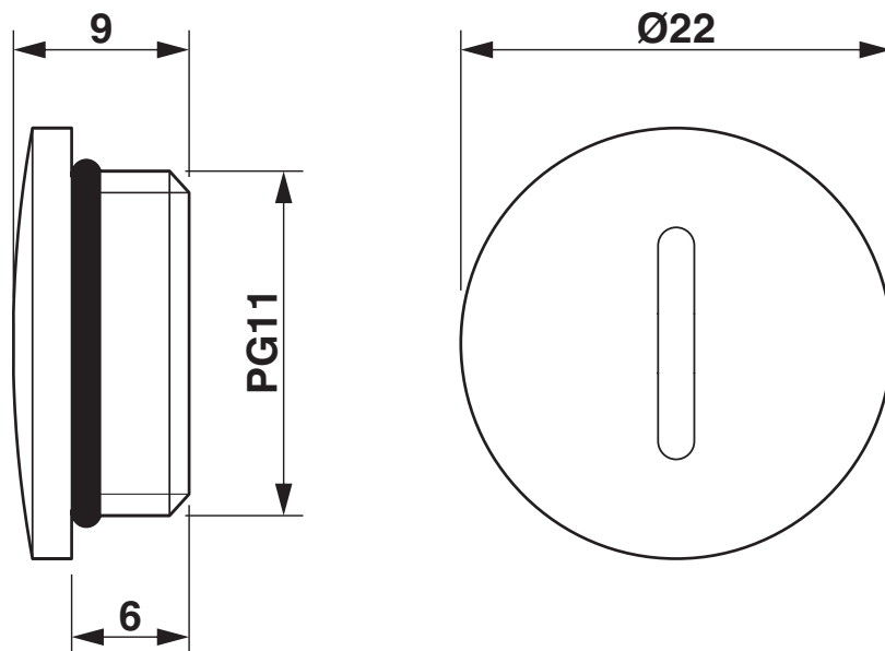
Rysunek wymiarowy
