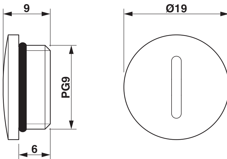
Rysunek wymiarowy
