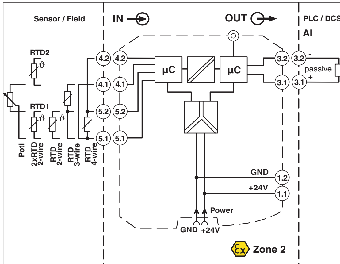
Schemat blokowy
