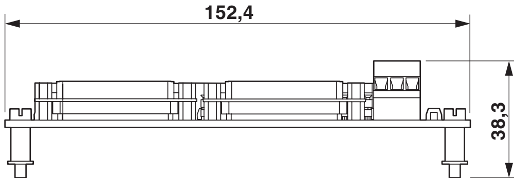
Rysunek wymiarowy
