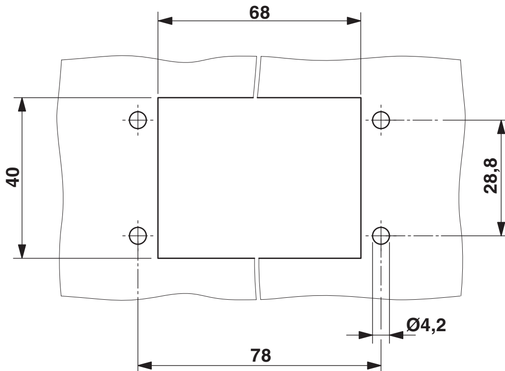
Rysunek wymiarowy
