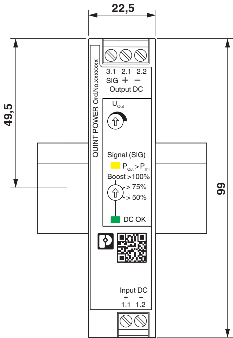
Rysunek wymiarowy
