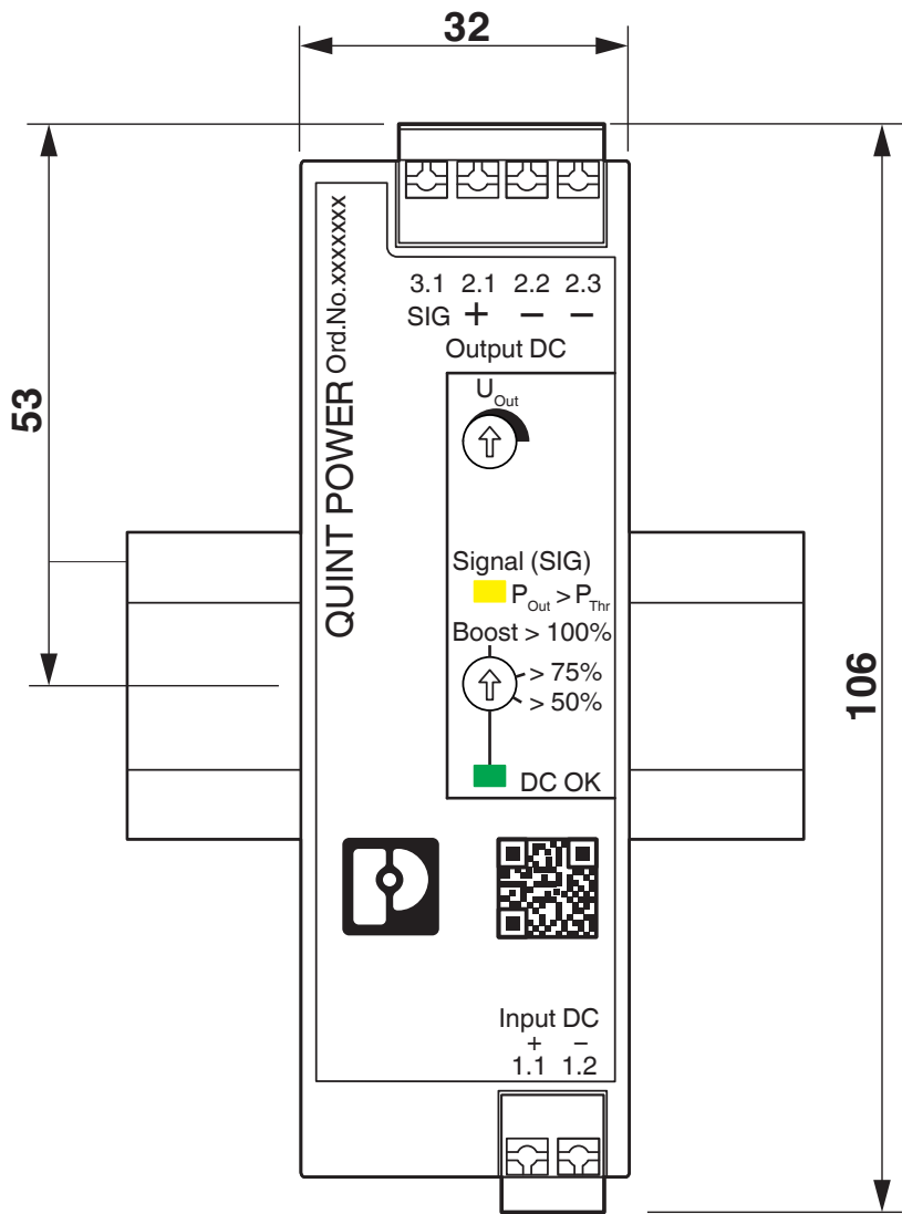
Rysunek wymiarowy
