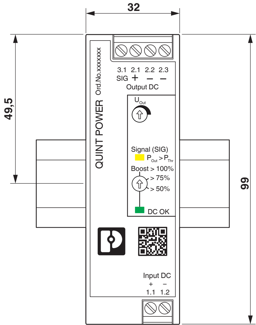
Rysunek wymiarowy
