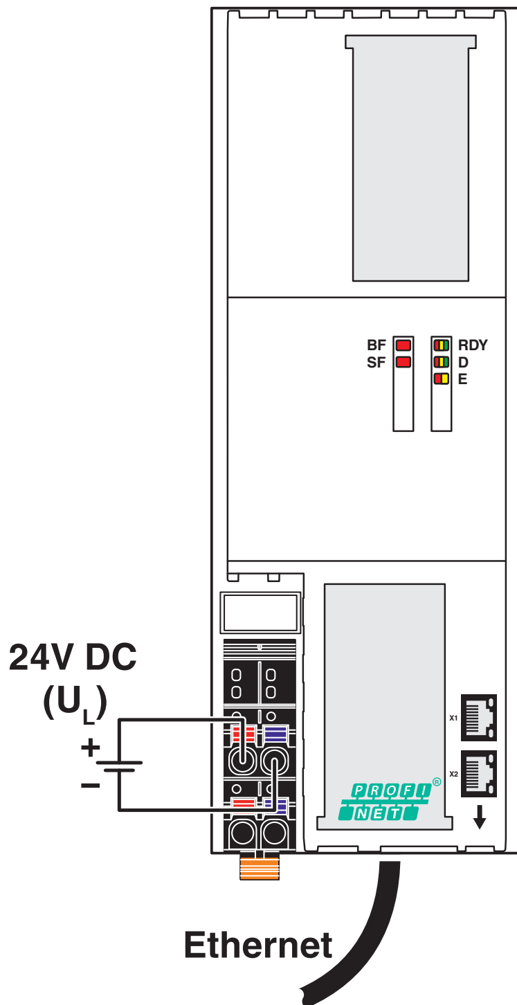
rysunek złączy
