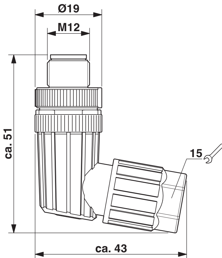
Rysunek wymiarowy
