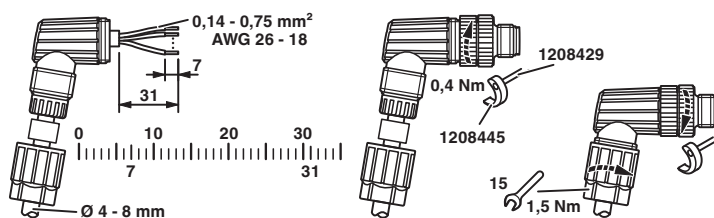
rysunek funkcyjny
